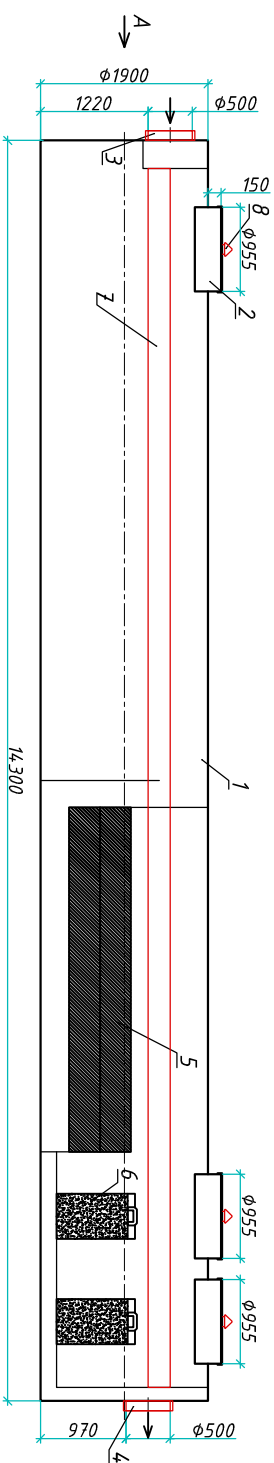
Разрез 1-1
