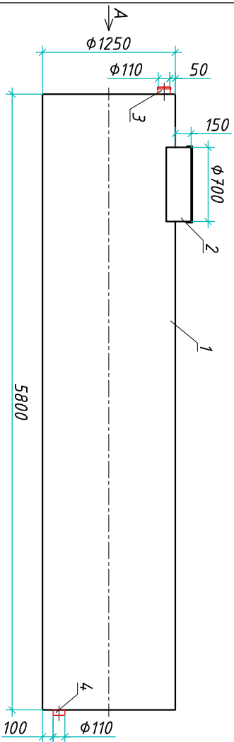
Разрез 1-1
