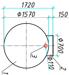
Вид А
