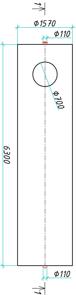
Вид сверху
