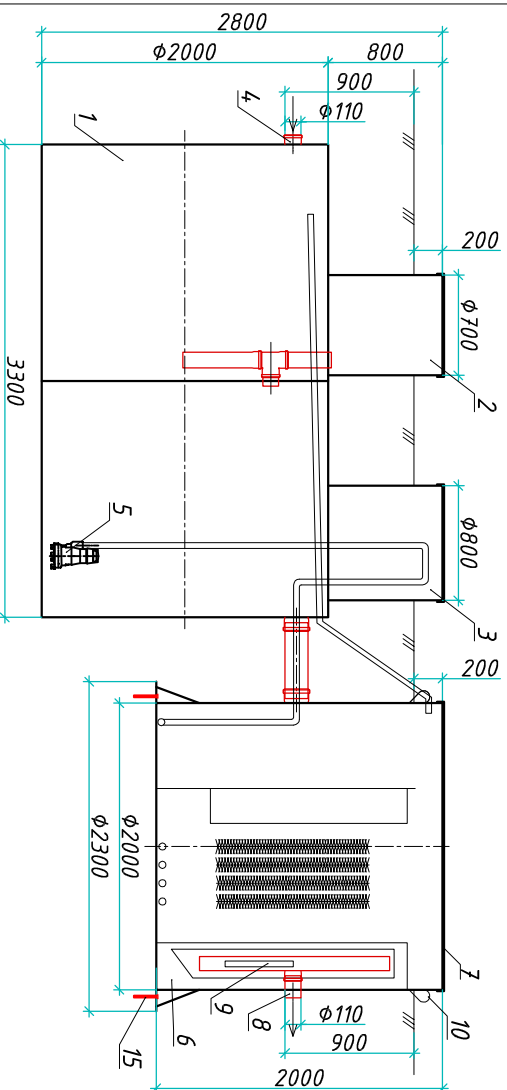
Разрез 1-1
