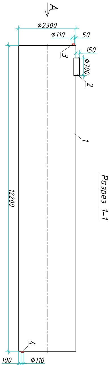
Разрез 1-1
